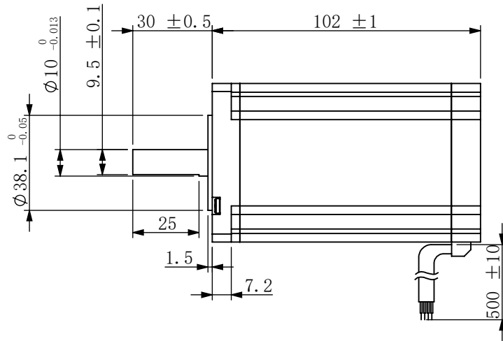
步 距 角/STEP ANGLE 1.8° ±5% 相 数/NO. OF PHASES 2 额定电压/RATED VOLTAGE 2.6V 额定电流/RATED CURRENT 5.0A 电 阻/RESISTANCE 0.52ohm±10% AT25℃ 电 感/INDUCTANCE 1.75mH±20% AT 1kHz, 1Vrms 保持力矩/HOLDING TORQUE 4.0N.m 运行力矩/(AT —PPS) RUNNING TORQUE(AT —PPS) ——以上/MIN (——V.DC, ——A/相(PHASE), ——相励磁/EX) 绝缘耐压/DIELECTRIC STRENGTH 500V A.C 1分钟/MINUTE 绝缘电阻/INSULATION RESISTANCE 100MΩ 以上/MIN. 绝缘等级/INSULATION CLASS CLASS B 温度上升/TEMPERATURE RISE 80K MAX. 转子惯量/ROTOR INERTIA 880g.cm 2 重 量/WEIGHT 约/APPROX. 2050克/g 允许轴向负载/ALLOWABLE THRUST LOAD 5N 允许径向负载/ALLOWABLE RADIAL LOAD 30N(轴端/ON THE SHAFT END) 运行环境温度/OPERATION AMBIENT TEMP. -20℃——+50℃ 运行环境湿度/OPERATION AMBIENT HUM. 15%——90%
