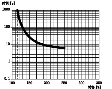
伺服电机的过载保护特性
