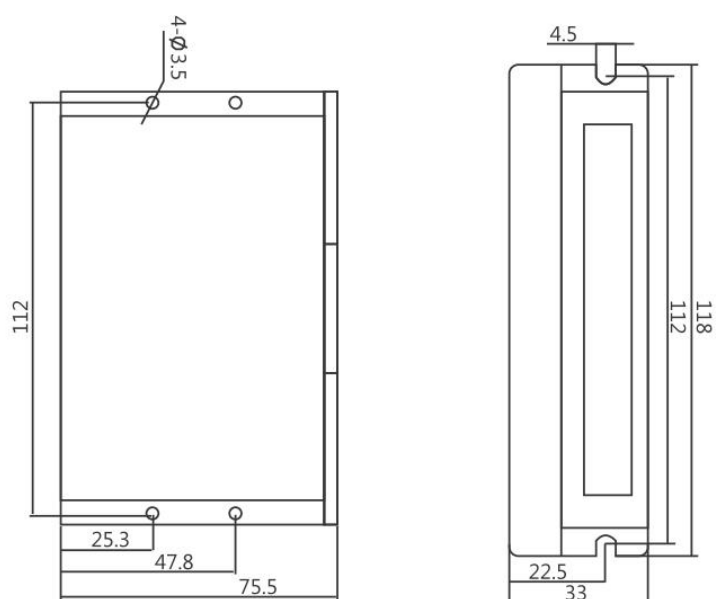
正面安装图
